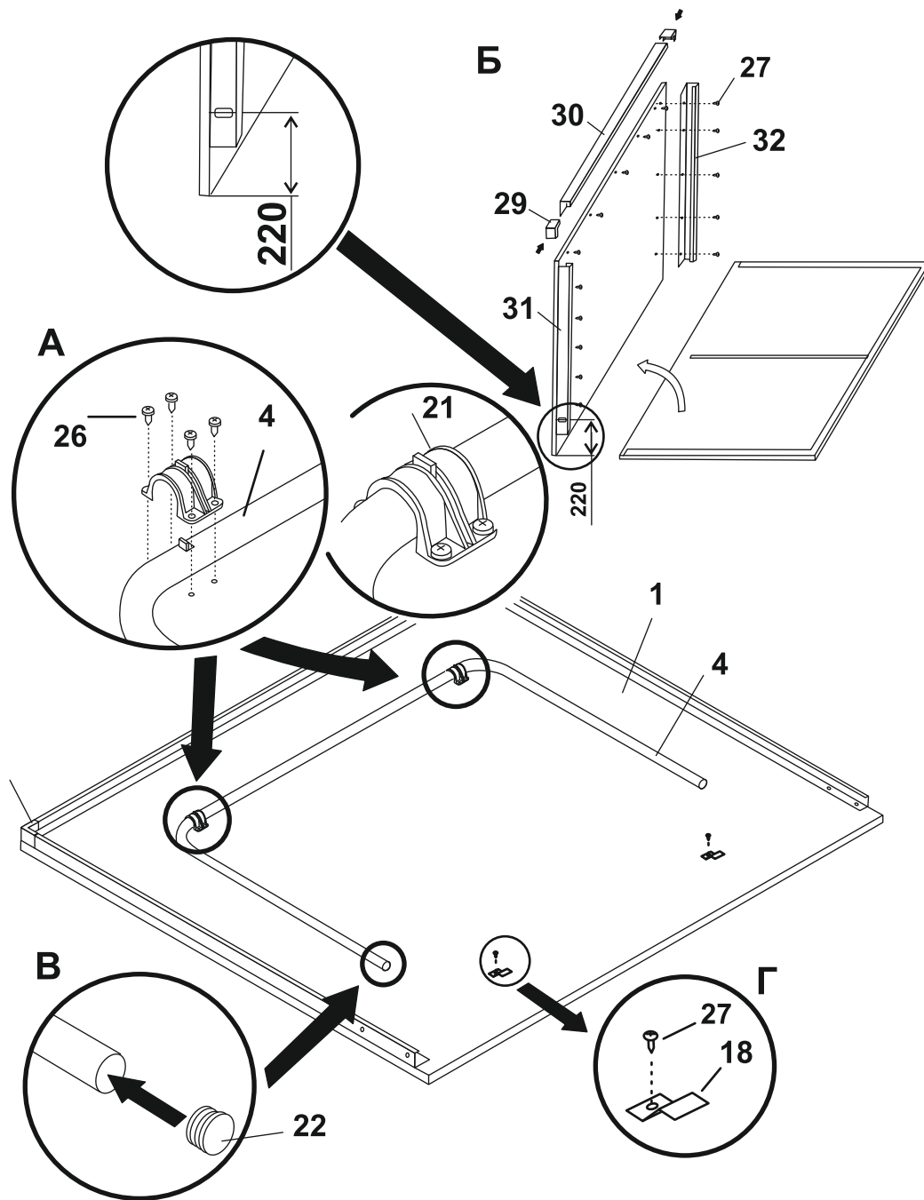
Сборка столешницы. Рис. 4
