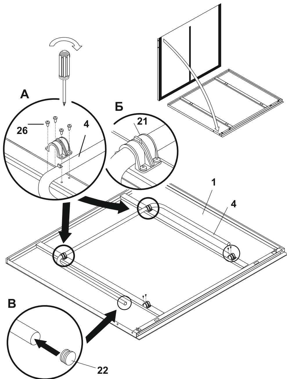
Сборка столешницы. Рис. 4
