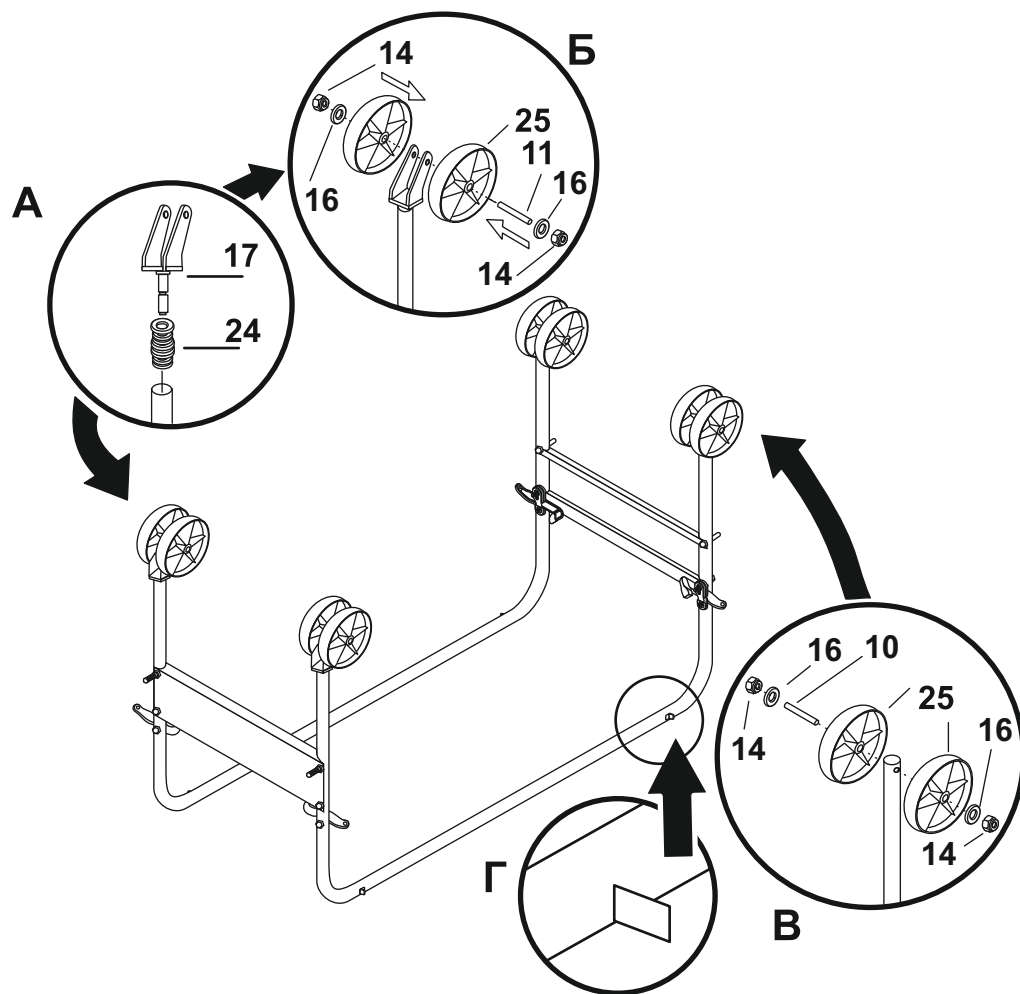
Сборка колес. Рис. 3
